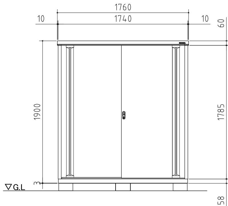
正面図
