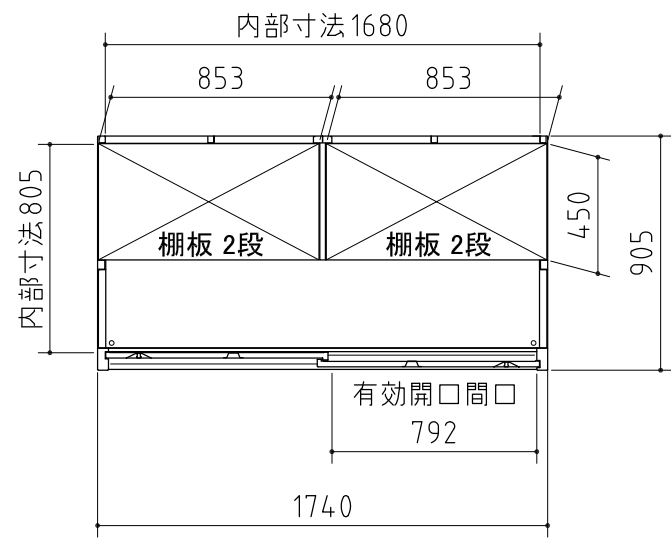
平面図
